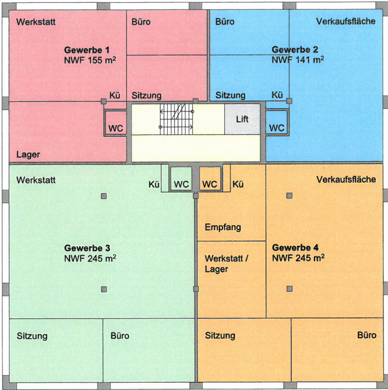
1./2. Obergeschoss Büro/ Werkstätten/KMU (Variante)
